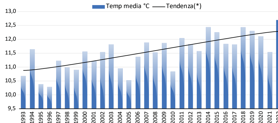
Andamento delle temperature medie annue calcolato sui dati relativi a 110 stazioni meteorologiche. Veneto – Anni 1993:2022
