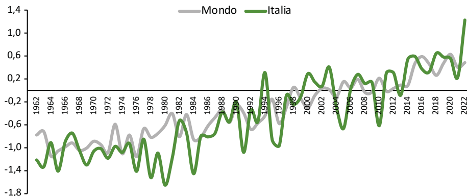
Serie delle anomalie medie annuali della temperatura media sulla terraferma, a livello mondiale e in Italia, rispetto ai valori climatologici standard del trentennio 1991-2020. Anni 1962:2022
